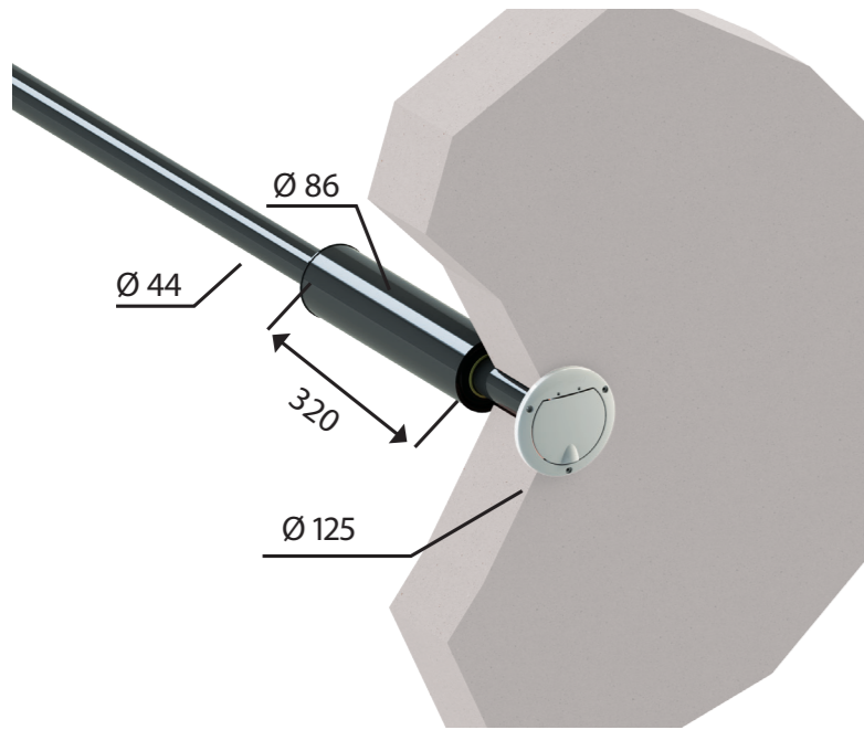
Bild 5. Der Schalldämpfer sollte so nahe wie möglich am Ende der Abluftleitung positioniert werden.
