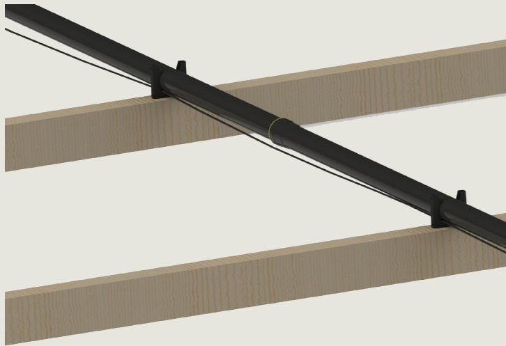
Bild 10. ALLWAY Rohrschellen fixieren die Rohre. Für die Steuerleitungen wurden in den Schellen Ausbuchtungen vorgesehen.
