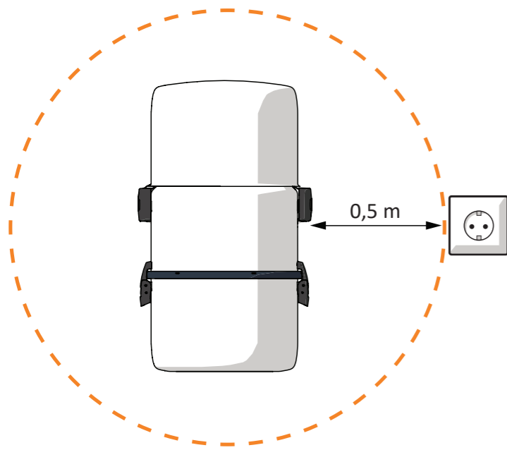
Bild 1. Montieren Sie eine Steckdose in der Nähe der Zentraleinheit.
