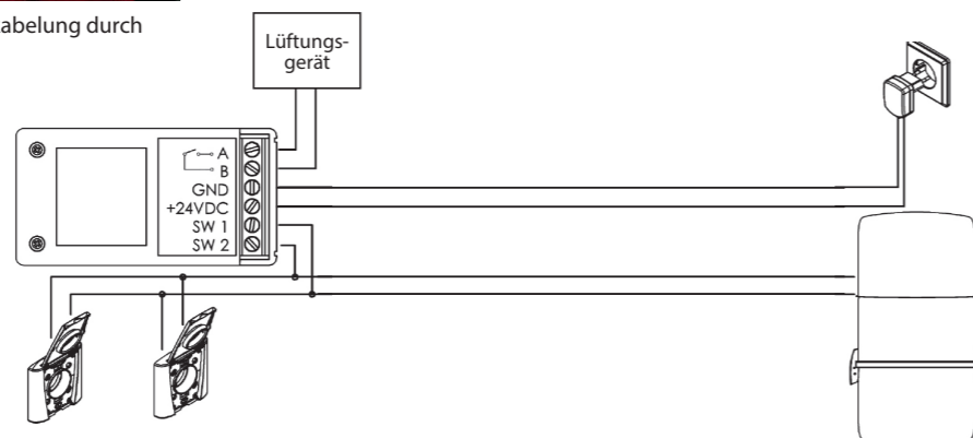
Bild 12. Beispiel einer Anwendung der Betriebsanzeige.
