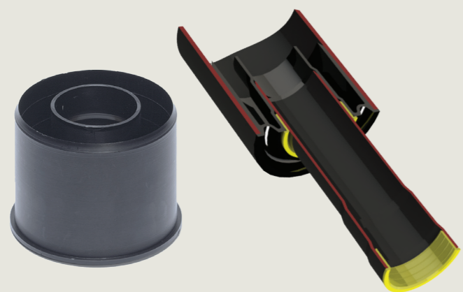
Bild 6. Eine Reduziermuffe 44/70/80 wird dann verwendet, wenn der Durchmesser der Abluftleitung aufgeweitet werden muss. Die Abluftleitung kann mit einem herkömmlichen glatten Rohr mit einem inneren Durchmesser von 75 mm aufgeweitet werden, wenn die Abluftlänge 5 m übersteigt.
