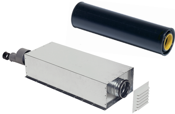
Bild 4. ALLAWAY bietet 2 Typen von Schalldämpfern. Der obere einfache Schalldämpfer reduziert den Lärmpegel um ca. 14 LpA (dB). Darunter der Turboschalldämpfer reduziert den Lärmpegel um ca. 20 LpA (dB).
