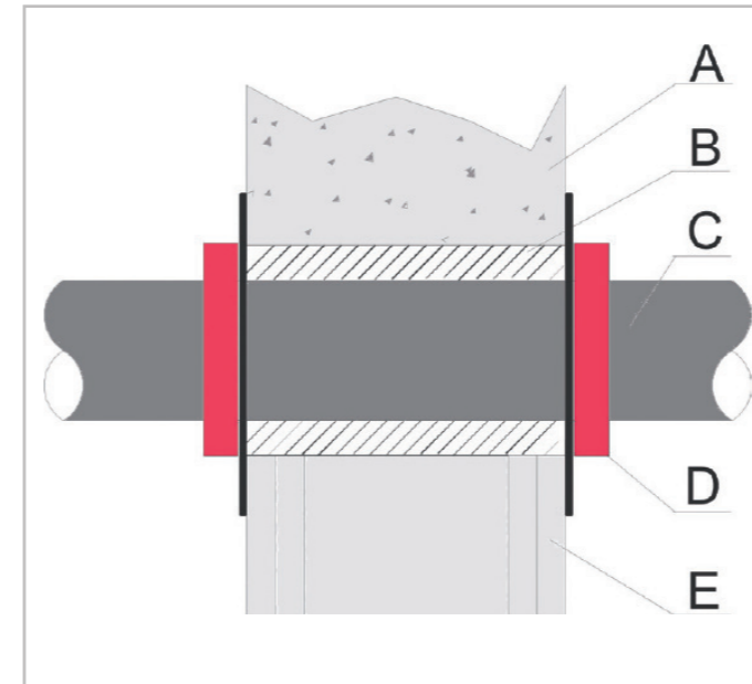
Bild 15. A Brandschutzwand
