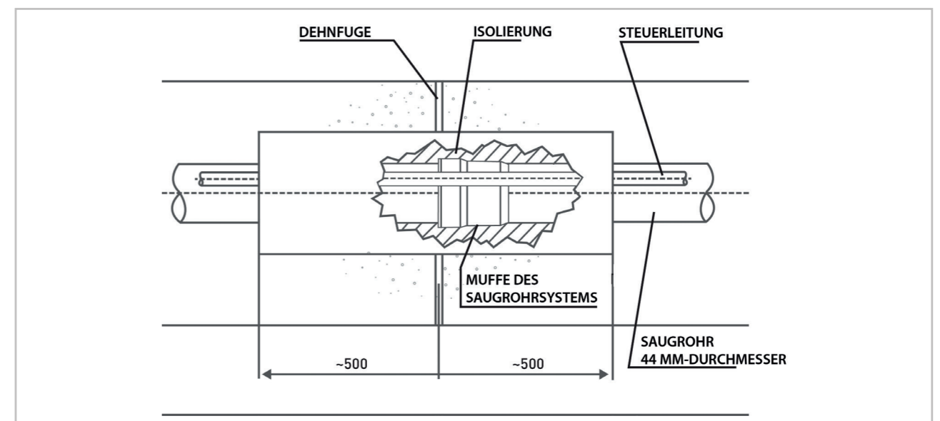
Bild 16. In gegossenen Bauteilen muss im Bereich der Dehnfuge das Rohr mit Schaumgummi isoliert werden.
