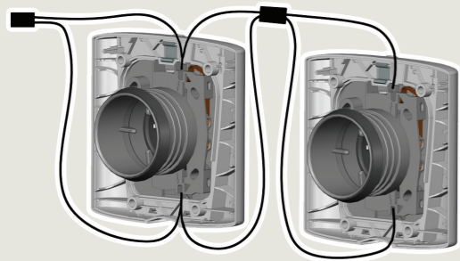
Bild 13. Parallelschaltung von Saugdosen
